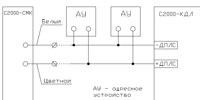
Рисунок 1 Схема соединений
