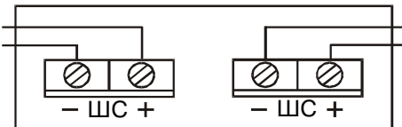
а) при включении в разрыв ШС
