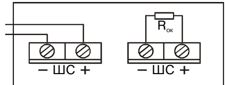
б) при включении на конце ШС
