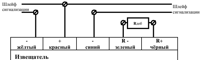
Рис. 1. Извещатель
