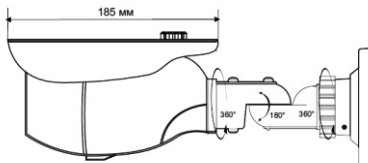
Рис.1 Вид сбоку
