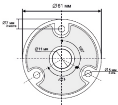
Рис.3 Крепежная платформа
