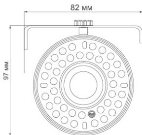
Рис.2 Вид спереди
