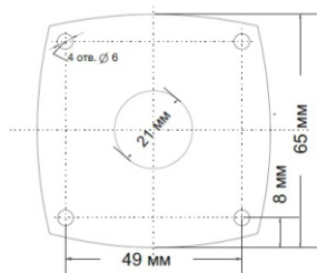
Рис.3 Крепежная платформа
