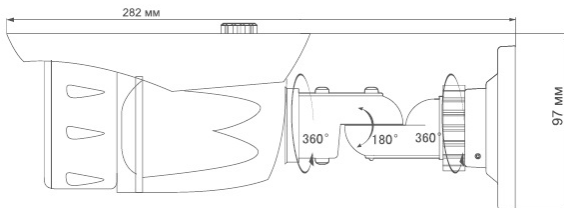
Рис.1 Вид сбоку
