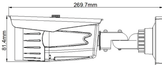
Рис.1 Вид сбоку
